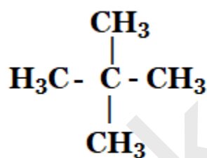
2,2 dimethylpropane
