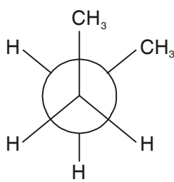
Gauche-conformer
